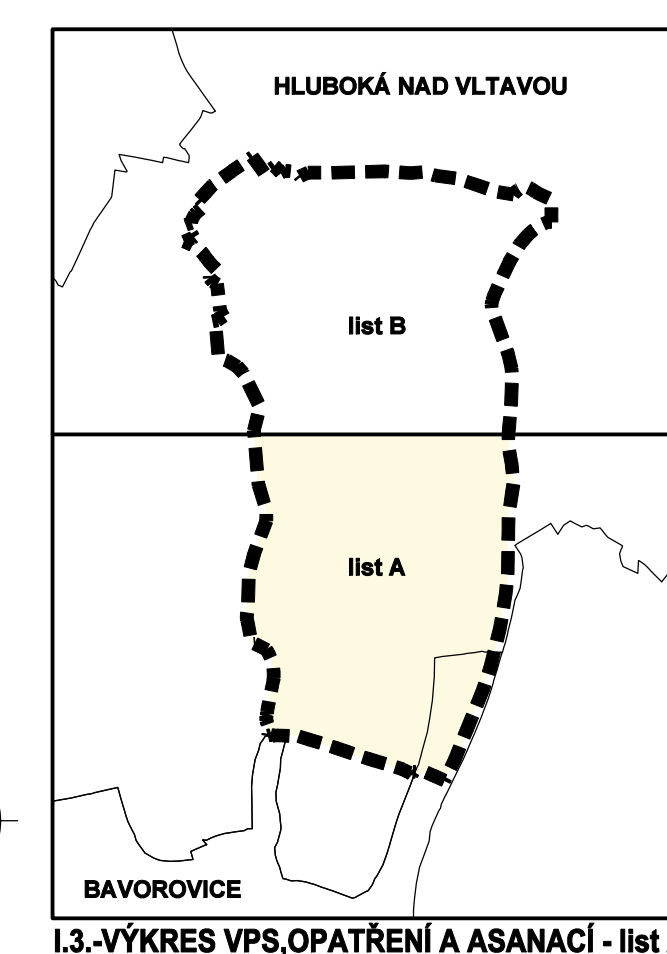
I.3.-VÝKRES VPS, OPATŘENÍ A ASANACÍ - list A
